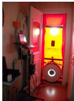
Réalisation du test d'étanchéité - Mai 2013
